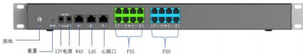
图 2: UCM6308 后面板接线图
