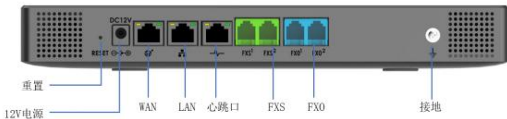
图 1: UCM6302 后面板接线图
