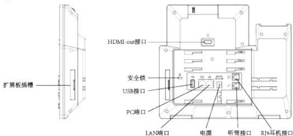
图 1: GXV3350 背面及侧面图
