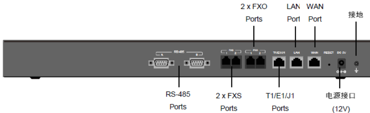
图 3: HA100 后面板
