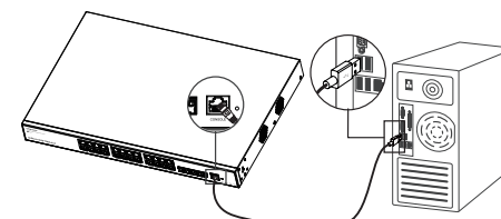
Connexion au port console (USB)
