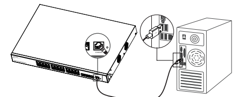
Anbindung über den Konsole-Port (USB)
