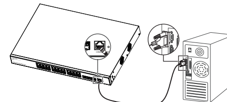
Anbindung über den Konsole-Port (DB9)
