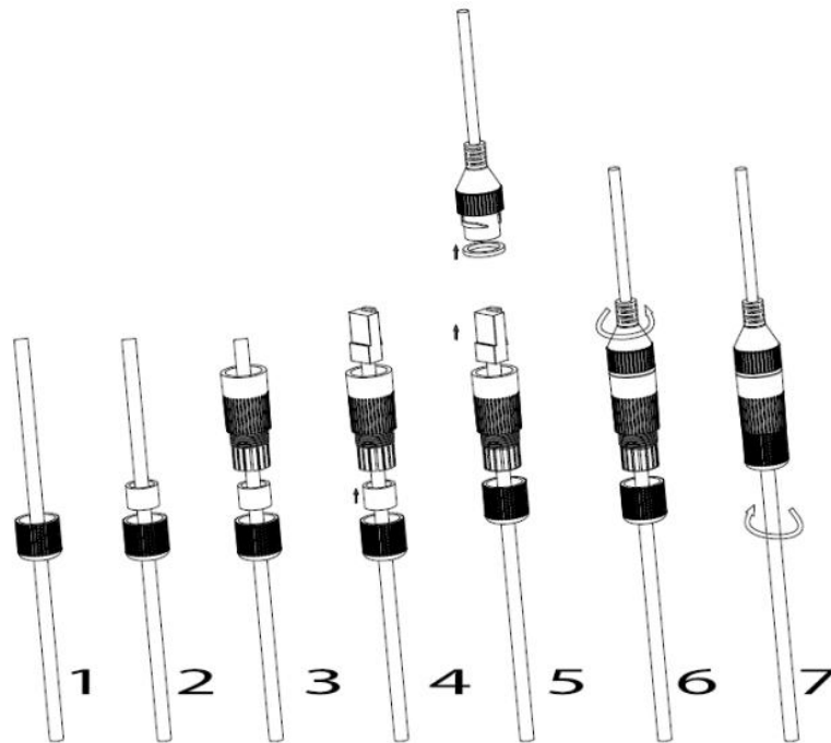
图 2 连接示意图
